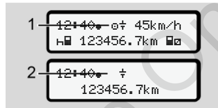
Joon. 129: Näit - toitepinge viga
