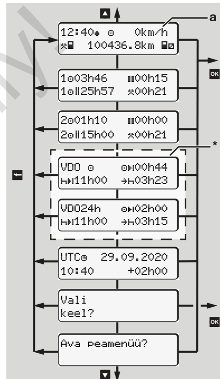
Joon. 59: Esimene menüütasand (*= valikuline VDO Counter)
