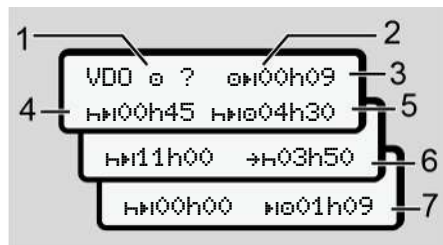
Joon. 62: VDO Counter - näidu ehitus
