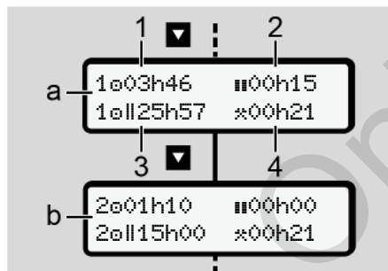
Joon. 60: Andmed juhikaardilt 1 või 2
