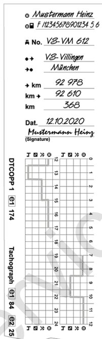
Joon. 31: Tegevuste käsikirjaline registreerimine
