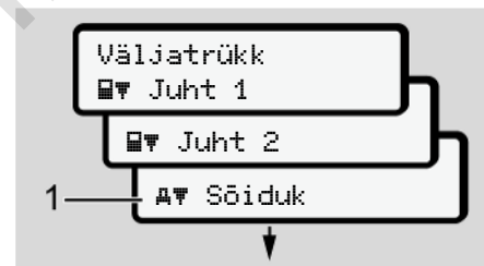
Joon. 78: Lehitsemine (põhi-)menüüs
