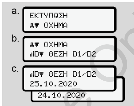
Εικ. 96: Αλληλουχία μενού εκτύπωσης - Κατάσταση D1/D2
