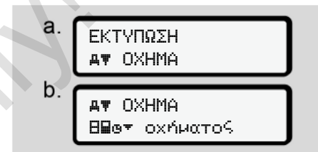
Εικ. 94: Αλληλουχία μενού εκτύπωσης - Πληροφορίες καρτών ταχογράφου
