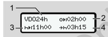
Εικ. 73: Ενέργεια * / - Τιμές ημέρας
