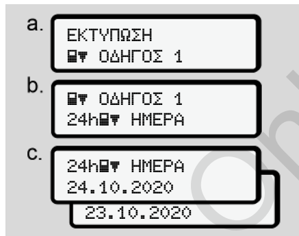
Εικ. 86: Αλληλουχία μενού εκτύπωσης – Τιμή ημέρας για τον Οδηγό 1
