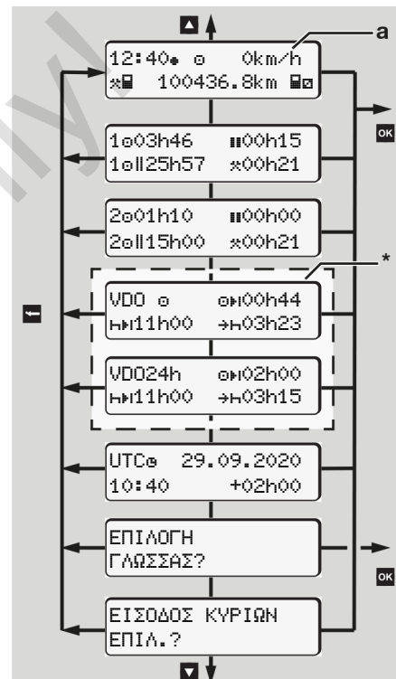
Εικ. 59: Πρώτο πεδίο μενού (*=Επιλογή μετρητή VDO)
