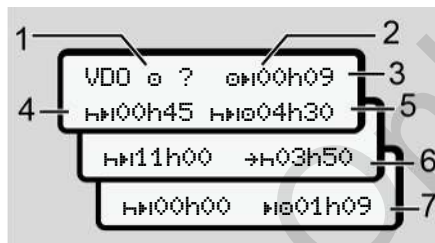
Εικ. 62: Μετρητής VDO - Δομή της ένδειξης
