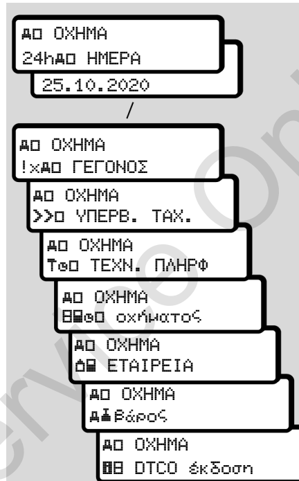
Εικ. 115: Αλληλουχία μενού Ένδειξη για όχημα
