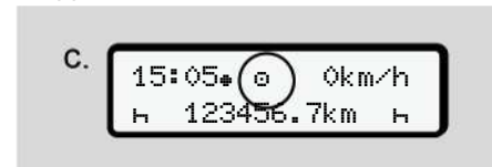
Рис. 56: Стандартная индикация без карт DTCO 4.1x снова находится в режиме «Эксплуатация», символ ⊙ .
