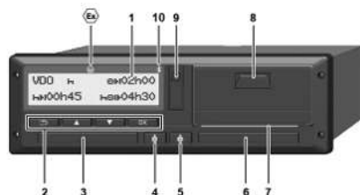
Рис. 1: Вид спереди DTCS 4.1x
