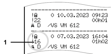
Obr. 144: Vysvětlivky ke kódování
