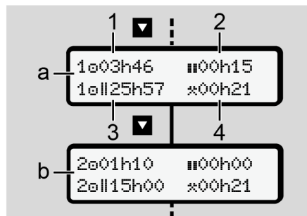
Obr. 58: Data z karty řidiče 1 nebo -2
