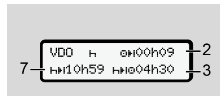
Obr. 68: Aktivita H – denní doba odpočinku
