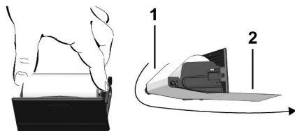
Obr. 142: Vložení role papíru
