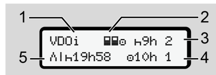
Obr. 74: VDO Counter – zobrazení stavu
