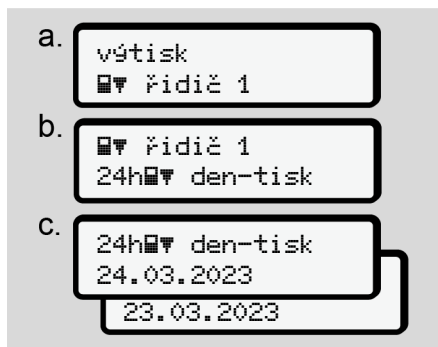
Obr. 84: Posloupnost výtisku – denní hodnota pro řidiče 1
