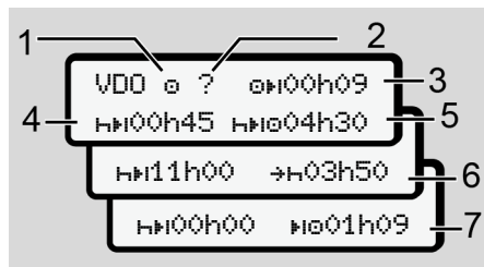
Obr. 60: VDO Counter – uspořádání displeje
