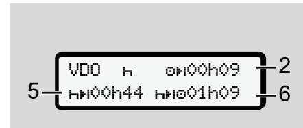
Obr. 67: Aktivita H – doba odpočinku vs. použitelná denní doba řízení
