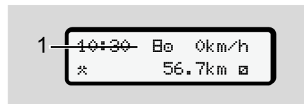
Obr. 133: Standardní zobrazení – stav výroby
