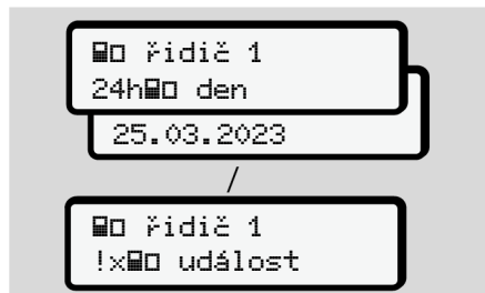
Obr. 126: Posloupnost zobrazení pro řidiče 1
