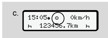
Obr. 32: Standardní zobrazení bez karet
