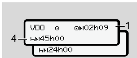
Obr. 63: Aktivita @ – zbývající doba řízení vs. týdenní doba odpočinku
