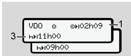
Obr. 62: Aktivita @ – zbývající doba řízení vs. denní doba odpočinku
