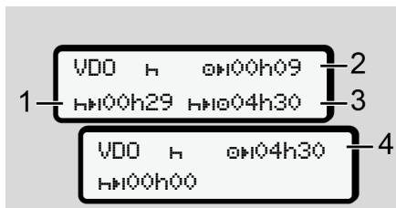
Obr. 66: Aktivita H – doba odpočinku vs. použitelná doba řízení
