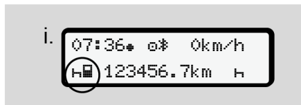
Obr. 23: Standardní zobrazení s vloženou kartou
