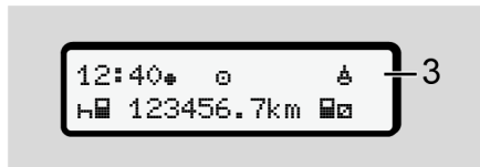
Obr. 135: Standardní zobrazení – trajekt/vlak
