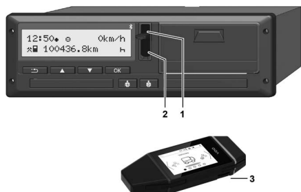
Obr. 12: Připojení k čelnímu rozhraní
