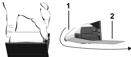
Рис. 142: Установка рулона бумаги
